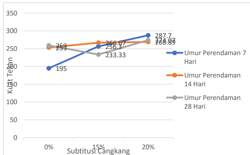
Gambar 2. Perbandingan Substitusi Cangkang Kerang Sebagai Agregat Halus
