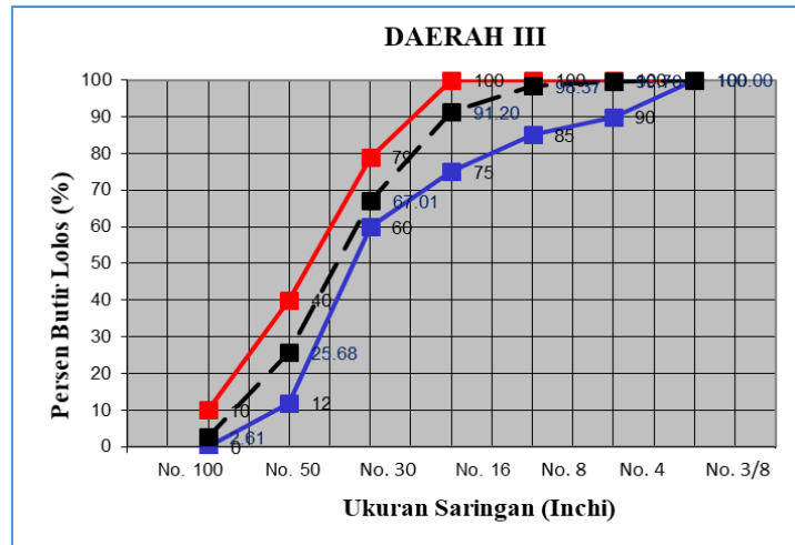
Gambar 1. Grafik Gradasi Agregat Halus
