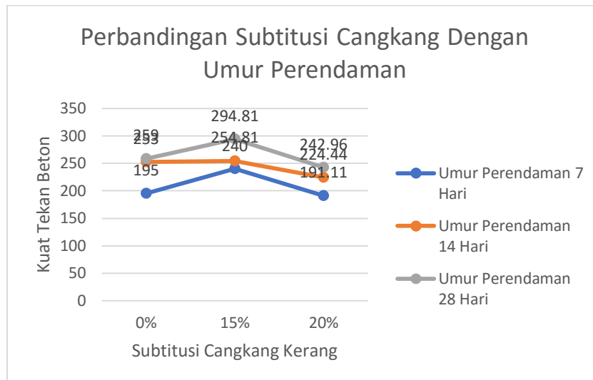
Gambar 3. Grafik Perbandingan substitusi cangkang kerang sebagai agregat kasar
