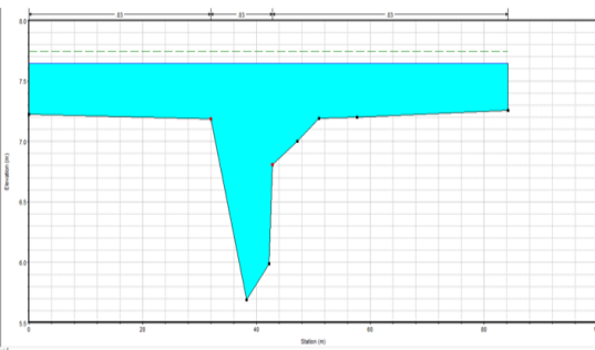
Gambar 4.4. Cross Section Sta 900
