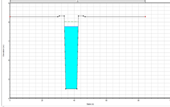
Gambar 4.13. Cross Section Sta 900 dengan Normalisasi dan Tanggul
