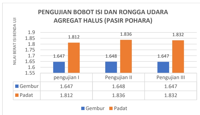
Grafik 3 Pengujian Bobot Isi dan Rongga Udara Pasir Pohara
