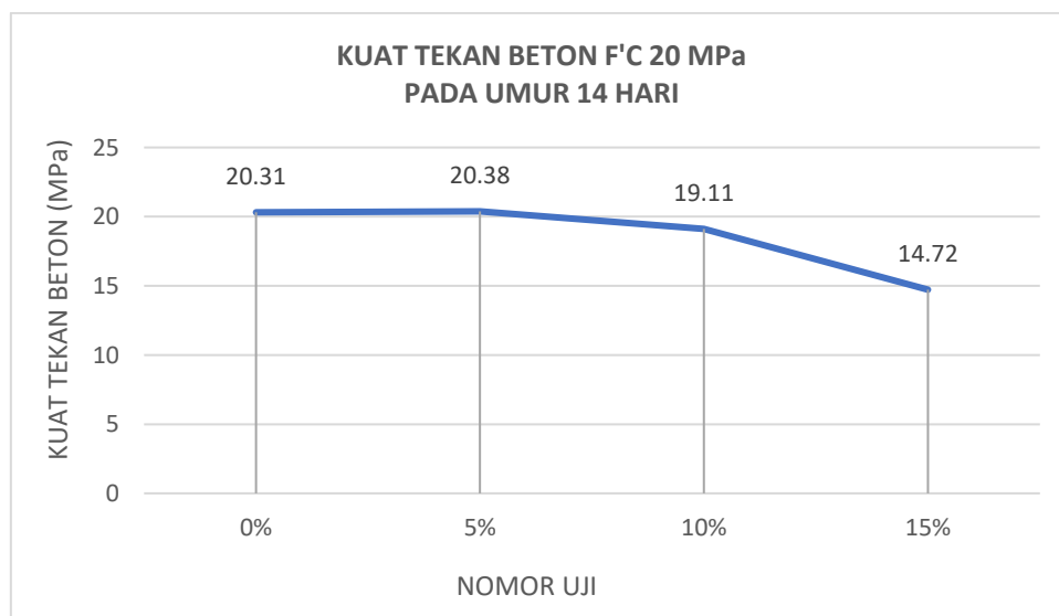
Grafik 7 Besar Kuat Tekan Beton Pada Umur 14 Hari
