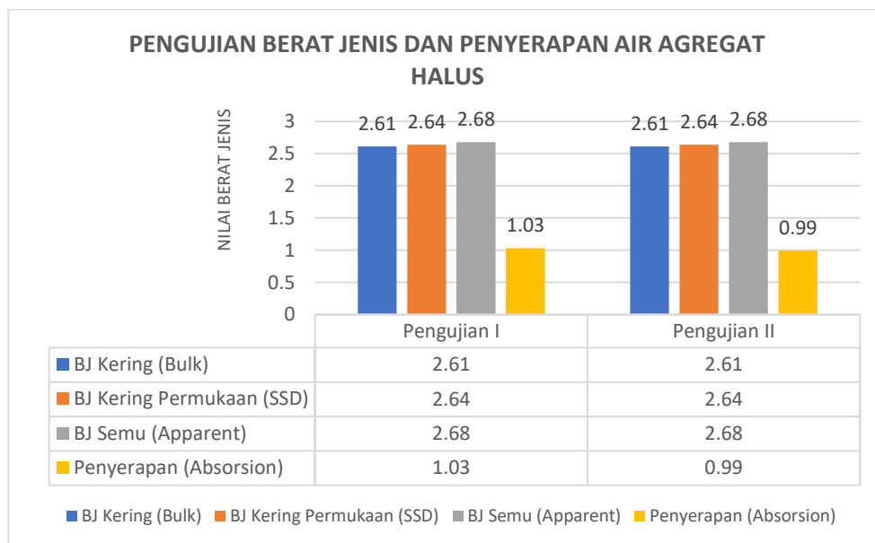
Grafik 4 Pengujian Berat Jenis Dan Penyerapan Air Pasir Pohara Sumber: Hasil Penelitian 2022
