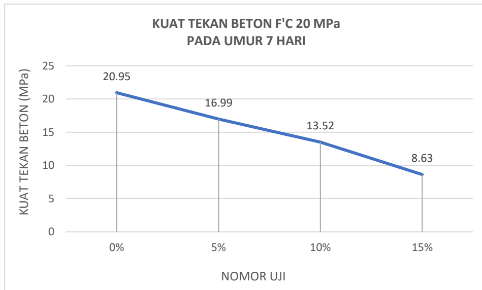
Grafik 6 Besar Kuat Tekan Beton Pada Umur 7 Hari
