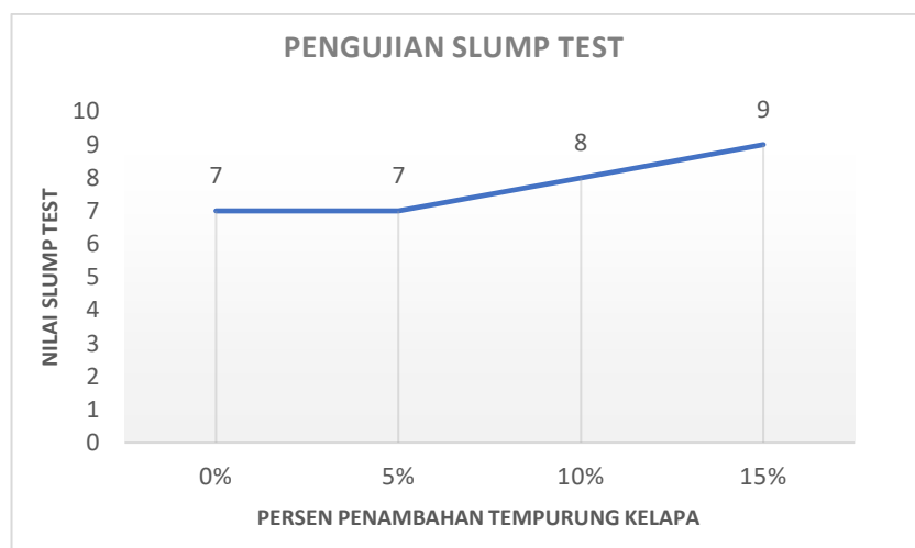
Grafik 5 Pengujian Slump Test Sumber: Hasil Penelitian 2022
